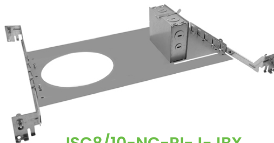
ISC8/10-NC-RI-J-JBX 18.5" W x 12" D x 4"H
