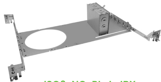
ISC6-NC-RI-J-JBX 18.5" W x 9" D x 4"H
